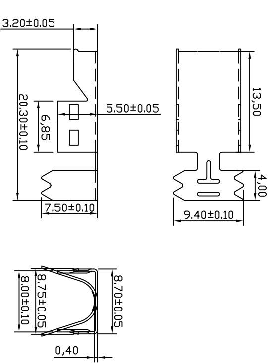
上铁壳
